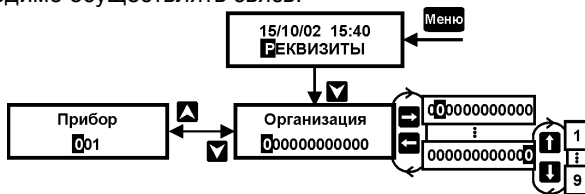
Рисунок 11 – Установка реквизитов
