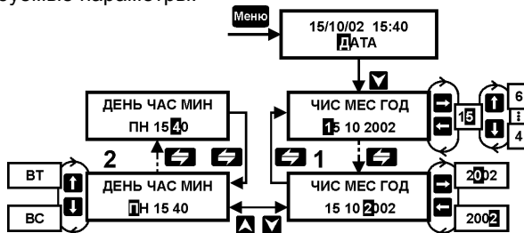
Рисунок 12 – Установка даты
